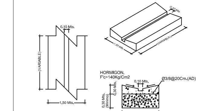
DETAILLE BADEN PLANTA & SECCION NO ESCALA
