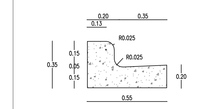
DETAILLE CONTEN SECCION NO ESCALA
